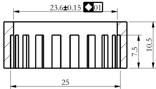
截面 A-A
